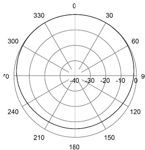
H-Plane | 98 MHz
