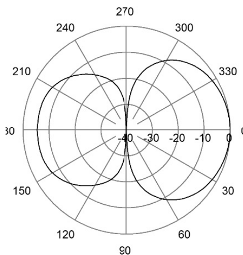
E-Plane | 225 MHz
