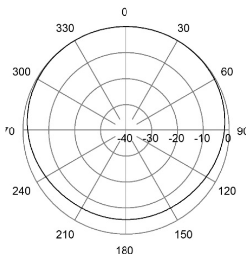
H-Plane | 225 MHz
