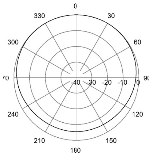
H-Plane | 459 MHz
