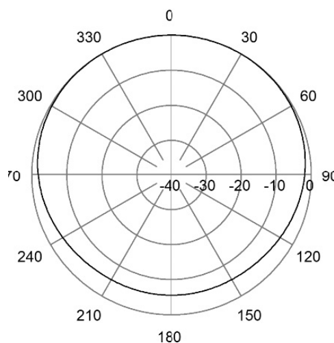
H-Plane | 405 MHz
