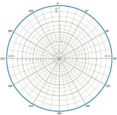
H-Plane | 132 MHz
